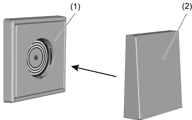
Bild 1: Lichtaufsatz montieren
