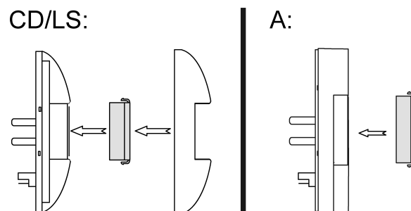
Bild 17: Montage Blende Programme LS/CD und A-Programme
