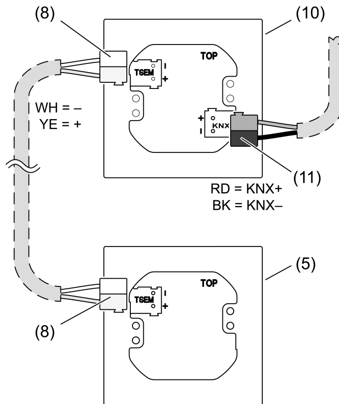
Bild 4: Anschluss Erweiterungsmodul
