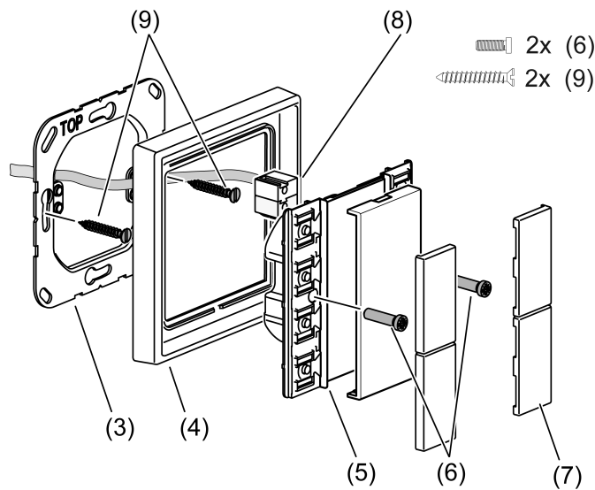
Bild 3: Montage Erweiterungsmodul
