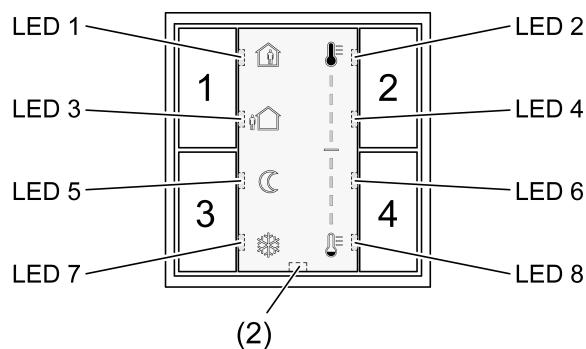
Bild 2: Raumcontroller-Erweiterungsmodule – Frontansicht
