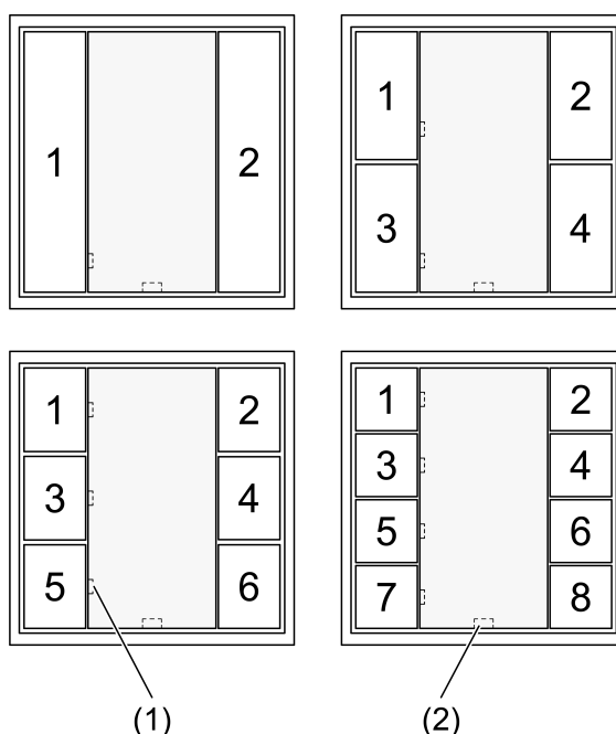
Bild 1: Tastsensor-Erweiterungsmodule – Frontansicht
