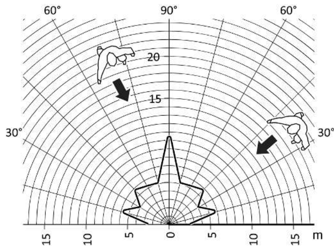
Bild 5: Reichweite bei radialer Bewegungsrichtung Bewegungsmelder 1,10 m Art.-Nr. ..17182..
